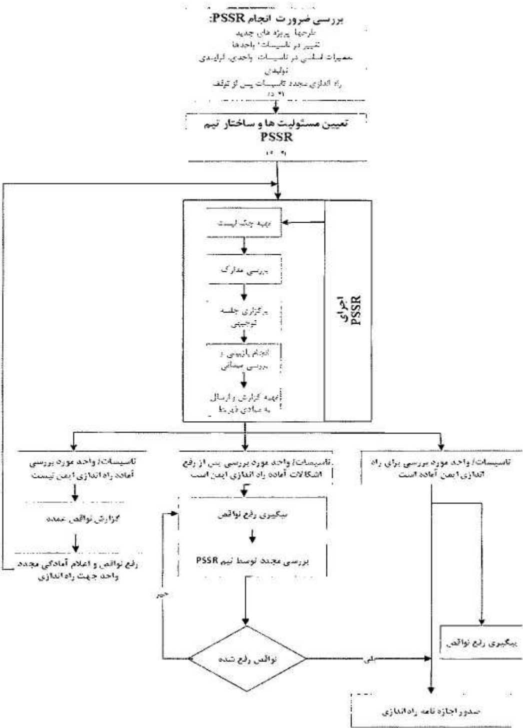
شکل شماره ۲: فلودیاگرام فرایند بازیابی ایمنی پیش از راه اندازی عملیاتی (PSSR)
